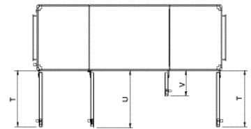
Вид сверху. Левосторонний агрегат
