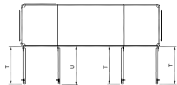
Вид сверху. Левосторонний агрегат
